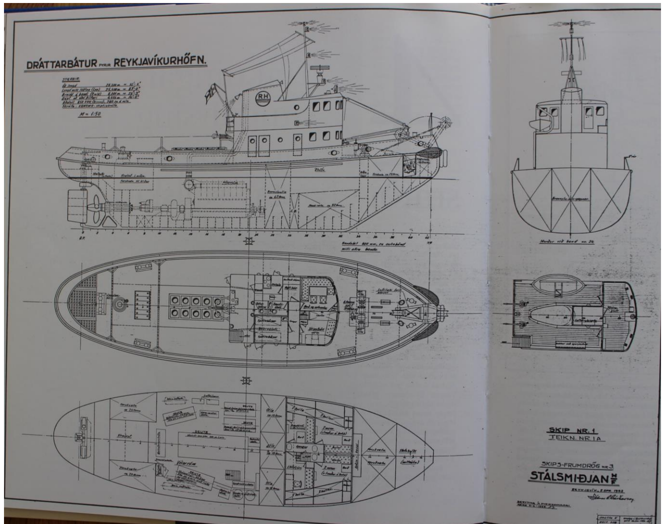
Teikning af ms Magna eftir Hjálmar R. Bárðarson, 1952. Teikningin er í bókinn Fyrsta stálskip smíðað á Íslandi e. Hjálmar .
