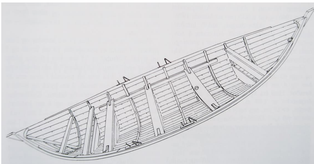
Teikning af Farsæli í Íslenskum sjávarhättum II, bls. 267.
